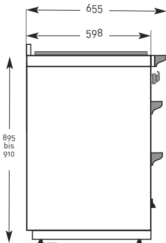
Sicht: seitlich/links
